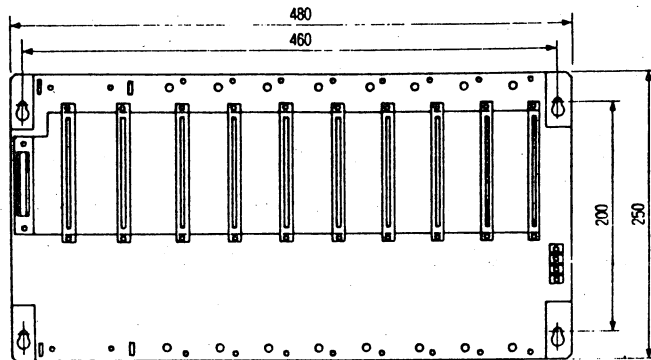
ZW-508KB CPU rack
