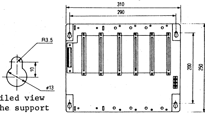
ZW-504KB CPU rack
