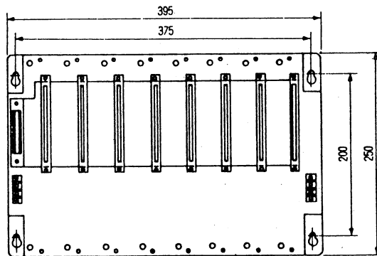
ZW-508ZB I/O rack
