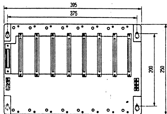
Expansion Rack Panel (ZW-508ZB)
