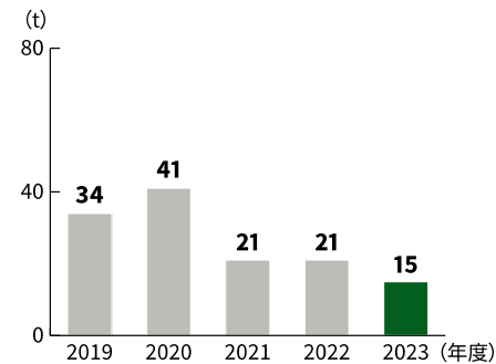
■ 窒素酸化物（NOx）排出量
