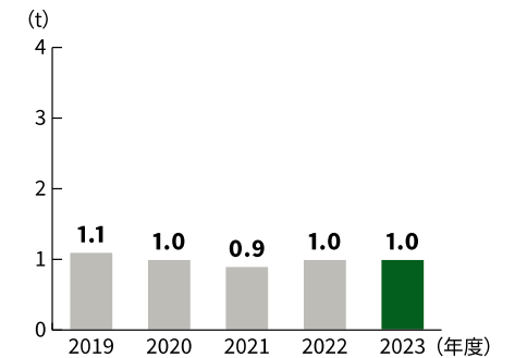
■ 硫黄酸化物（SOx）排出量
